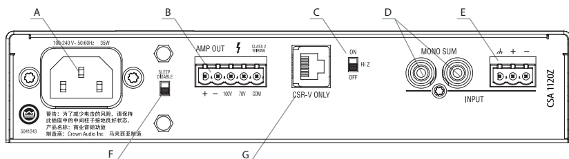
图 1.3 后面板 - CSA 1120Z
