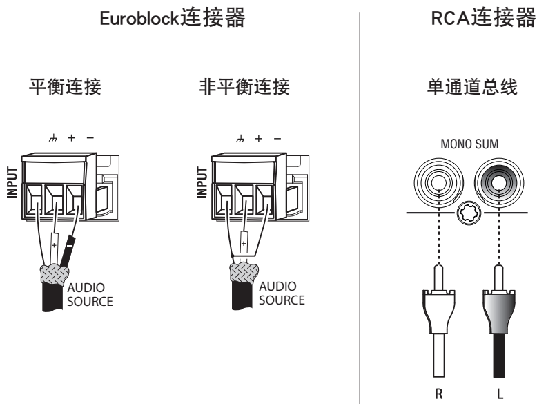
图2.4 输入连接
