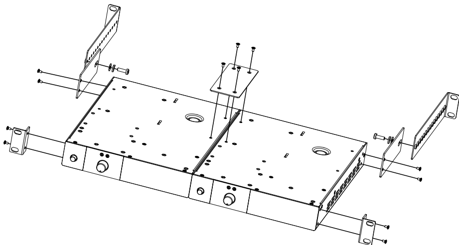
图2.2.3 安装两个功放到机柜
