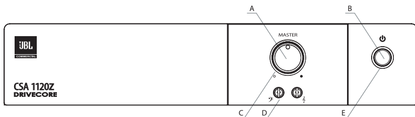
图 1.2 单通道的前视图
